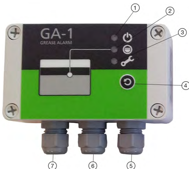
Afbeelding 2. Functies van regeleenheid GA-1
