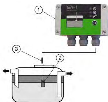
Afbeelding 1. Bewaking vetafscheider met alarmtoestel GA-1
