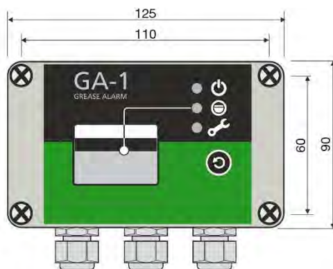
Afbeelding 7. Regeleenheid GA-1
