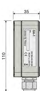
Afbeelding 7. Regeleenheid GA-1
