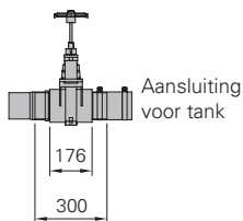
PVC-inlaatklep DN 100
