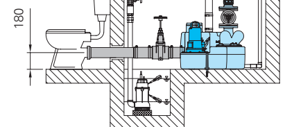
Directe aansluiting Euro-WC (toeloophoogte 180 mm)
