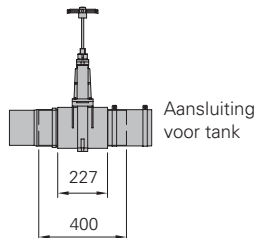
PVC-inlaatklep DN 150
