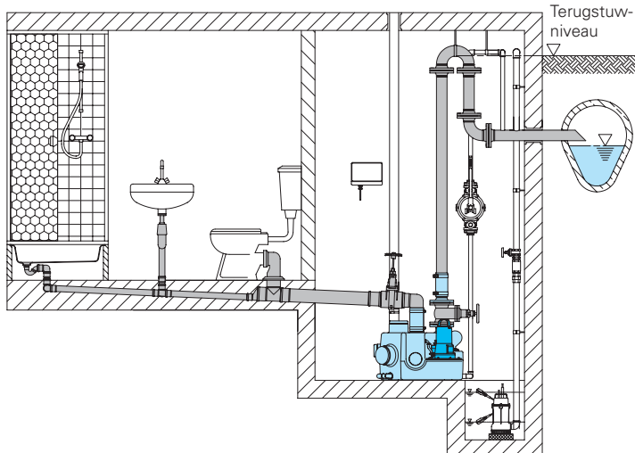
Hoofdtoeloop verticaal
