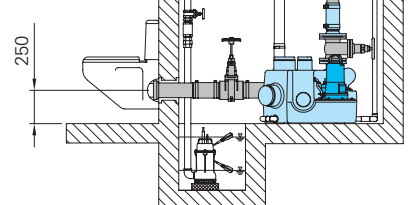
Directe aansluiting hangend toilet (toeloophoogte 250 mm)
